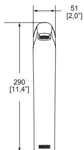
Dimensiones: vista frontal
