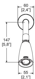
Dimensiones: vista frontal
