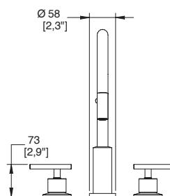
Dimensiones: vista frontal
