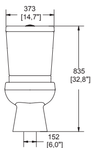
Dimensiones: vista frontal
