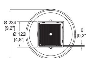
Dimensiones: vista cenital
