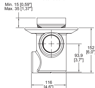
Dimensiones: vista lateral
