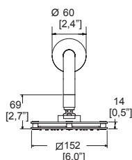
Dimensiones: vista frontal
