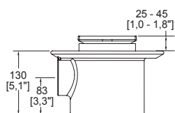
Dimensiones: vista lateral
