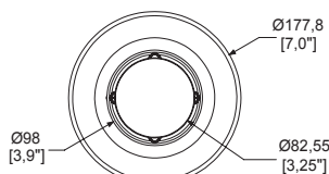
Dimensiones: vista cenital
