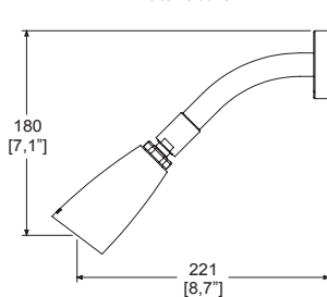
Dimensiones: vista lateral
