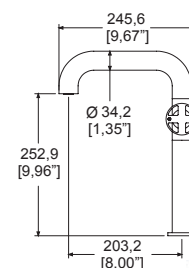
Dimensiones: vista lateral
