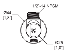
Dimensiones: vista frontal
