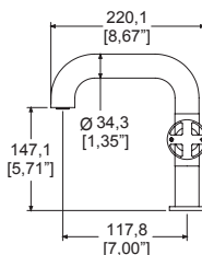
Dimensiones: vista lateral
