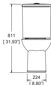
Dimensiones: vista frontal
