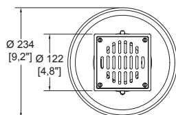
Dimensiones: vista cenital
